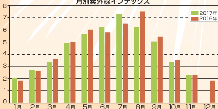
月別紫外線インデックス
